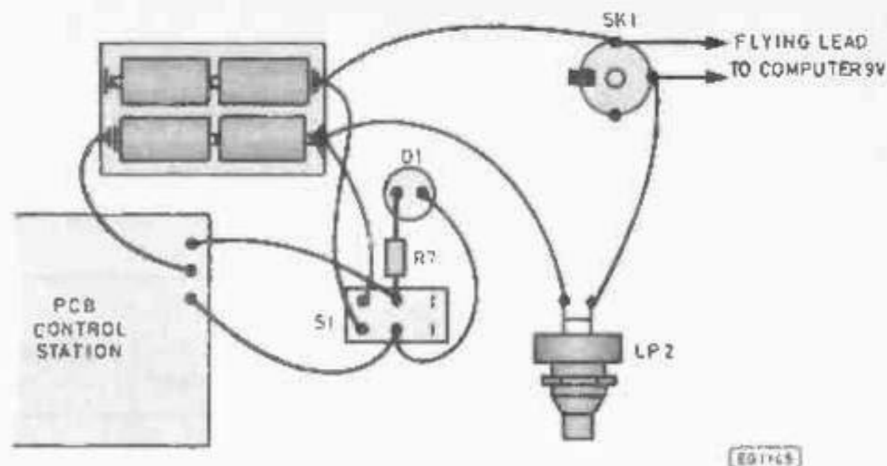
Fig. 4. Wiring diagram
